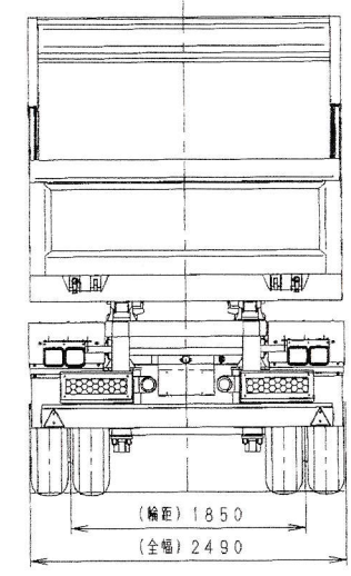
矢視 A-A
