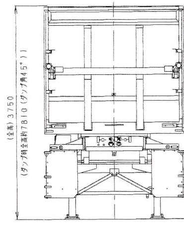
矢視 A-A
